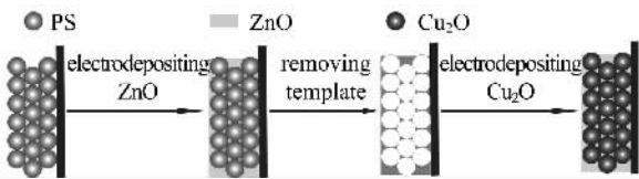
图 1 \text{Cu}_2\text{O} 与 ZnO 反蛋白石的复合材料制备过程的示意图 Fig. 1 Schematic diagram for synthesizing \text{Cu}_2\text{O} and ZnO inverse opal composite materials
