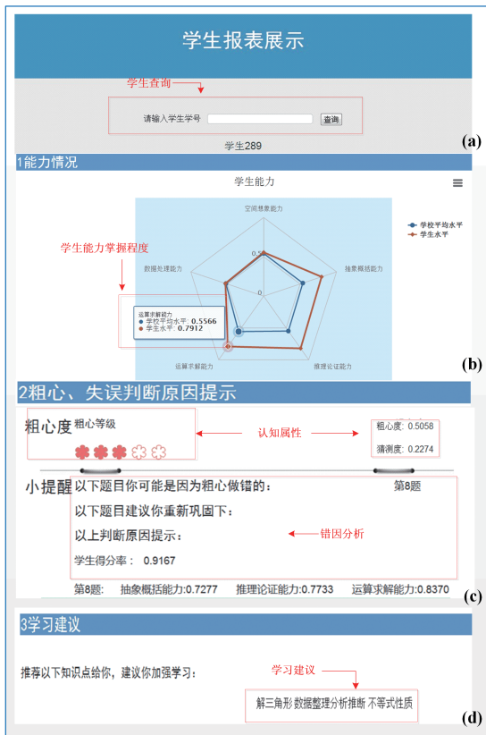
图 6 学生报表 Fig. 6 The student report
